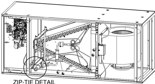
ZIP-TIE DETAIL
